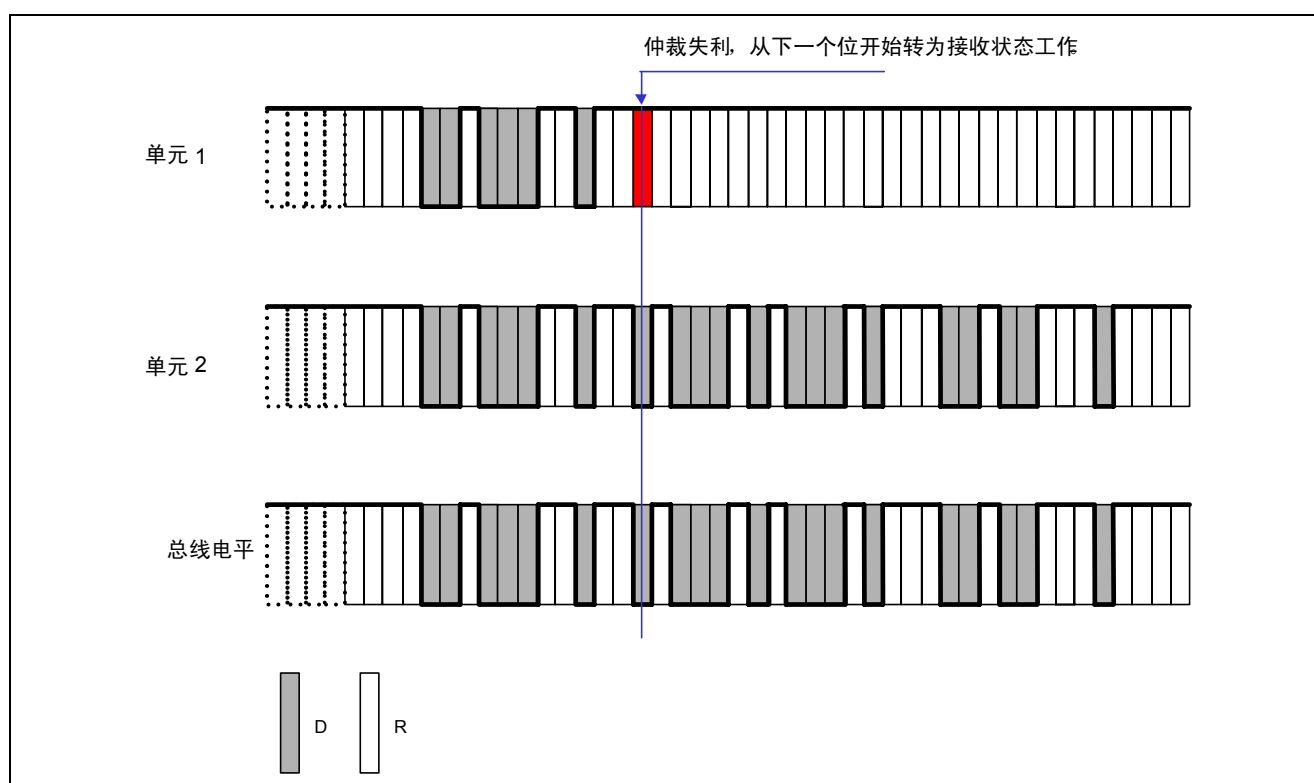
图 28. 仲裁过程
